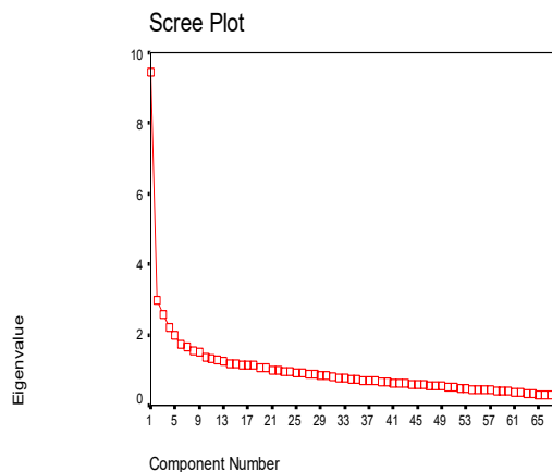
Slika 1 Grafički prikaz Scree plot testa
